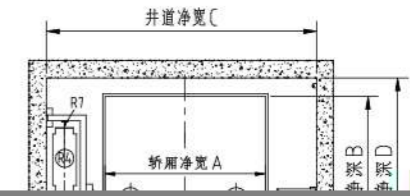
井道平面图 Hoistway plan
