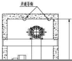
井道立面图 Hoistway elevation
