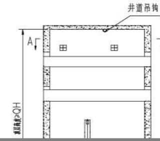
井道立面图 Hoistway elevation
